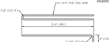
OPTIONAL LOOP DETAIL
