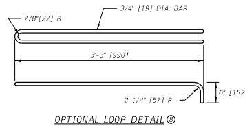
OPTIONAL LOOP DETAIL
