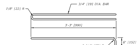
OPTIONAL LOOP DETAIL
