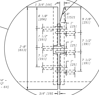
OPTIONAL TAPERED END
